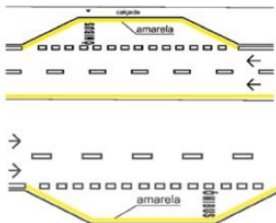
MARCA DELIMITADORA PARA PARADA DE ÔNIBUS FEITA EM REENTRÂNCIA DA CALÇADA
