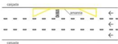
MARCA DELIMITADORA PARA PARADA DE ÔNIBUS FEITA EM REENTRÂNCIA DA CALÇADA
