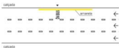
MARCA DELIMITADORA PARA PARADA DE ÔNIBUS EM FAIXA DE ESTACIONAMENTO
